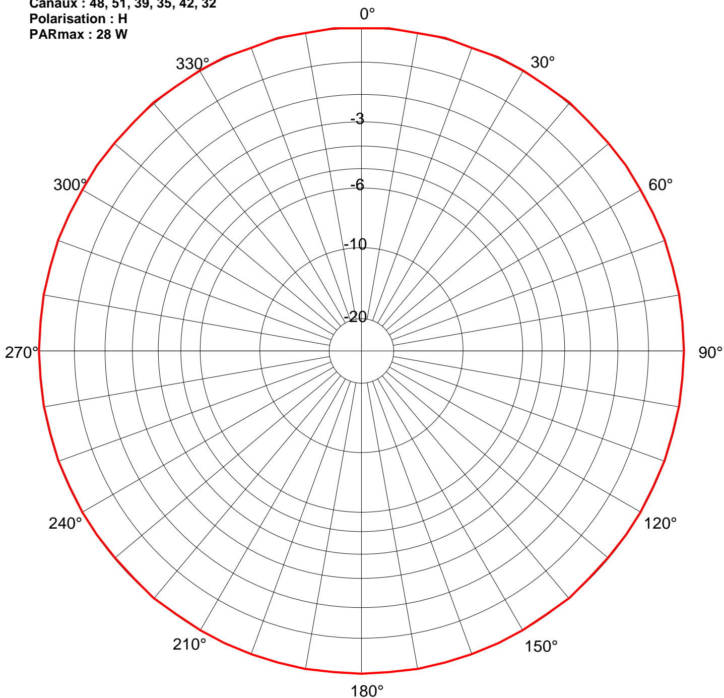
Diagramme omnidirectionnel
