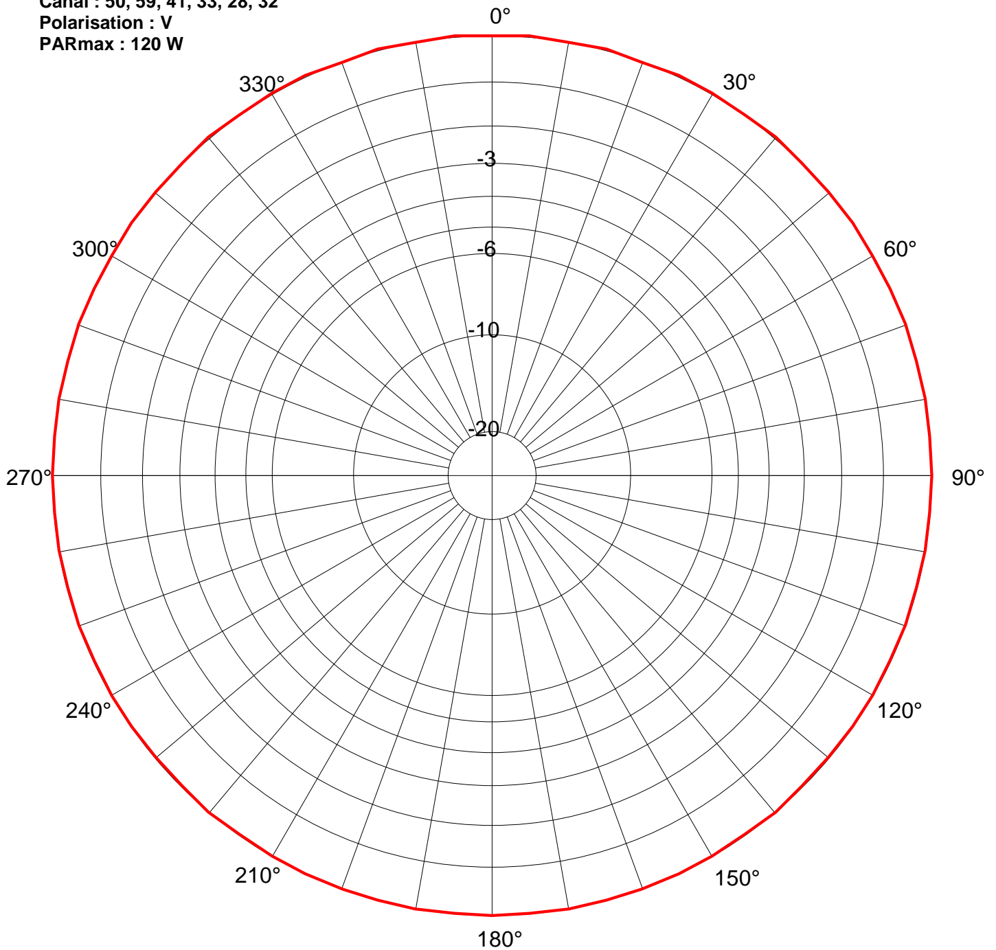
Diagramme omnidirectionnel
